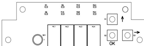
Рис. 4 Чертеж платы индикации и управления
