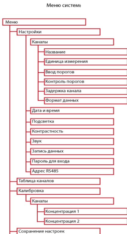
Рис. 14. Структура меню пульта контроля СККГ А-4М, СККГ А-8М
