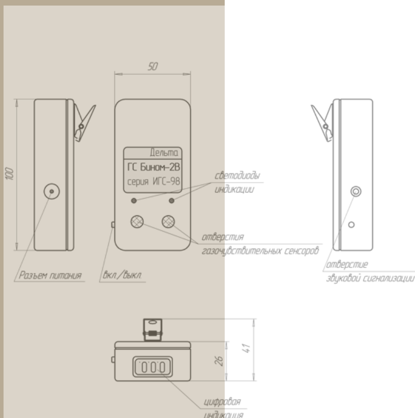
Габаритный чертеж
